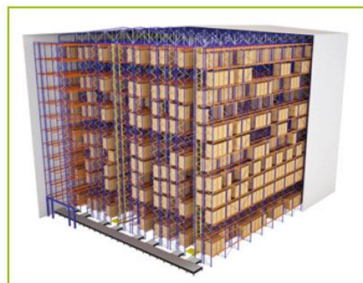
RAYONNAGE AUTOPORTANT
